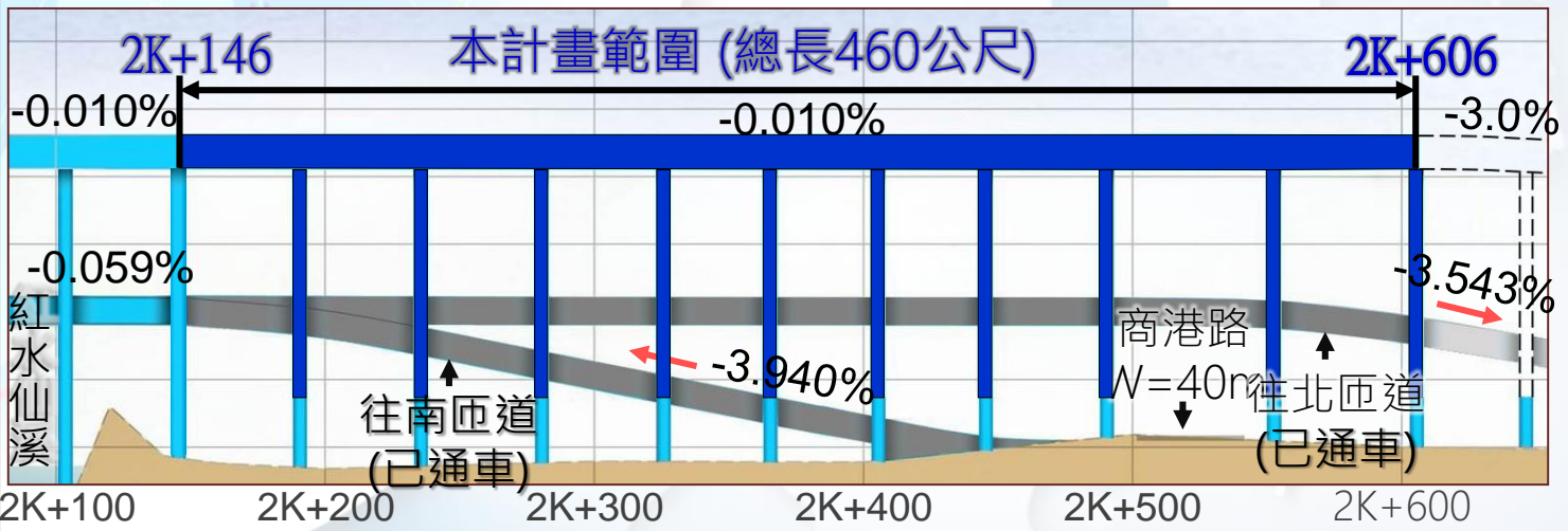
路線平縱斷面圖
